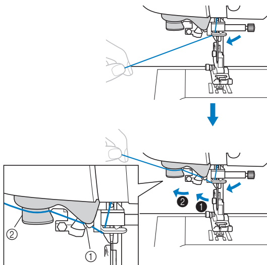
① Паз нитенаправителя нитевдевателя ② Нитенаправляющий диск нитевдевателя
